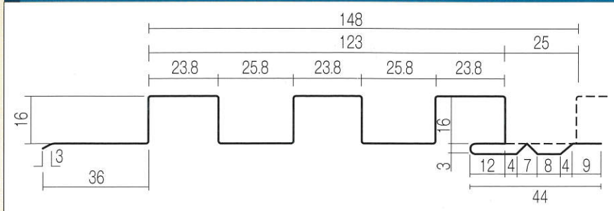
断面形状図
